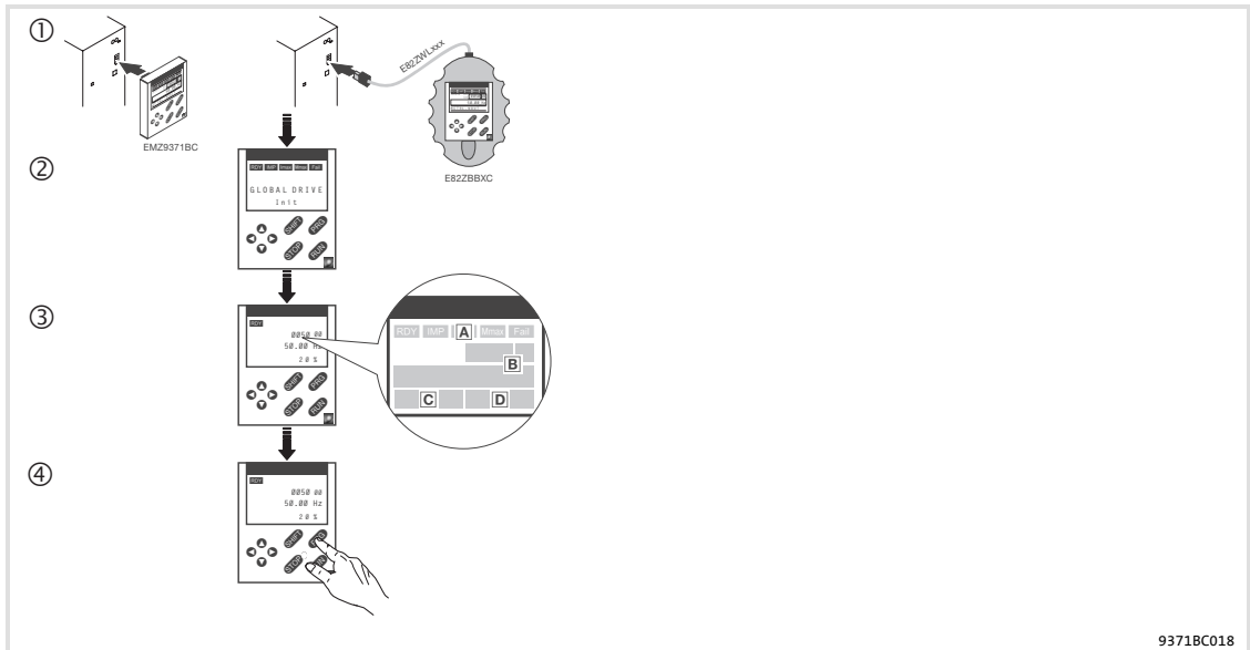
Abb. 2-1 Installation und Inbetriebnahme Keypad XT EMZ9371BC oder Handterminal E82ZBBXC
