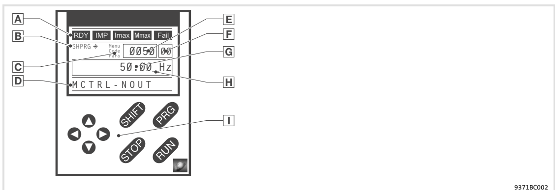
Abb. 2-2 Anzeige-Elemente und Funktionstasten Keypad XT EMZ9371BC
